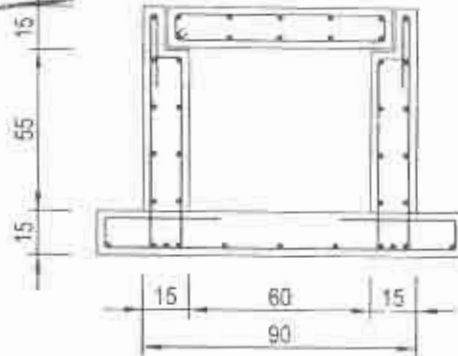
CANIVEAU DOUBLE
