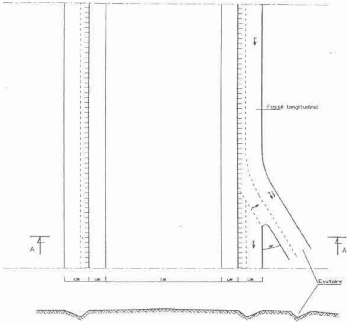
COUPE A-A
