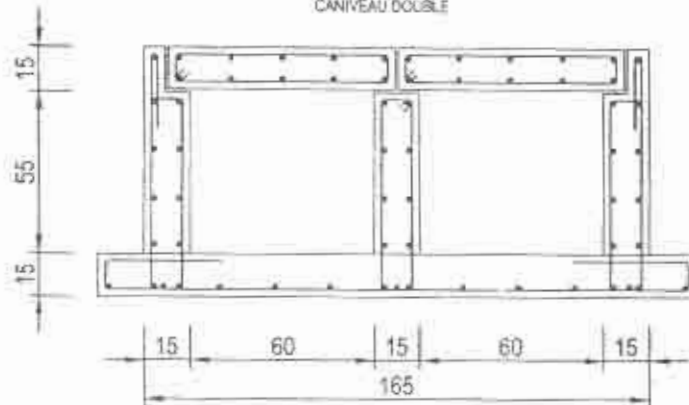
CANIVEAU DOUBLE
