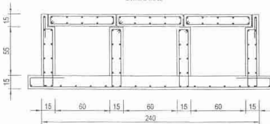
CANIVEAU TRIPLE
